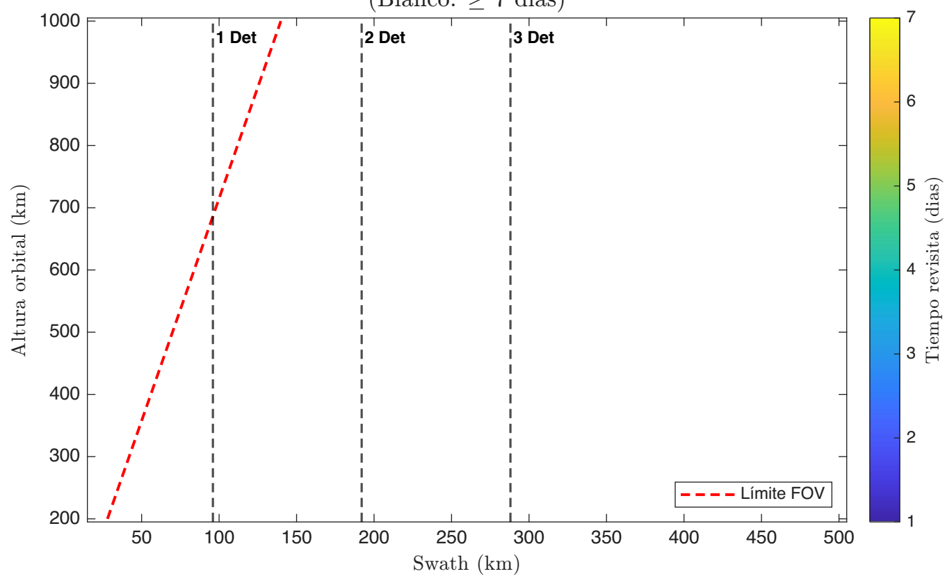
Tiempo Revisita - 2 Satelite(s); 1 Telescopio(s): TMA; Detector 1 (Blanco: \geq 7 dias)
